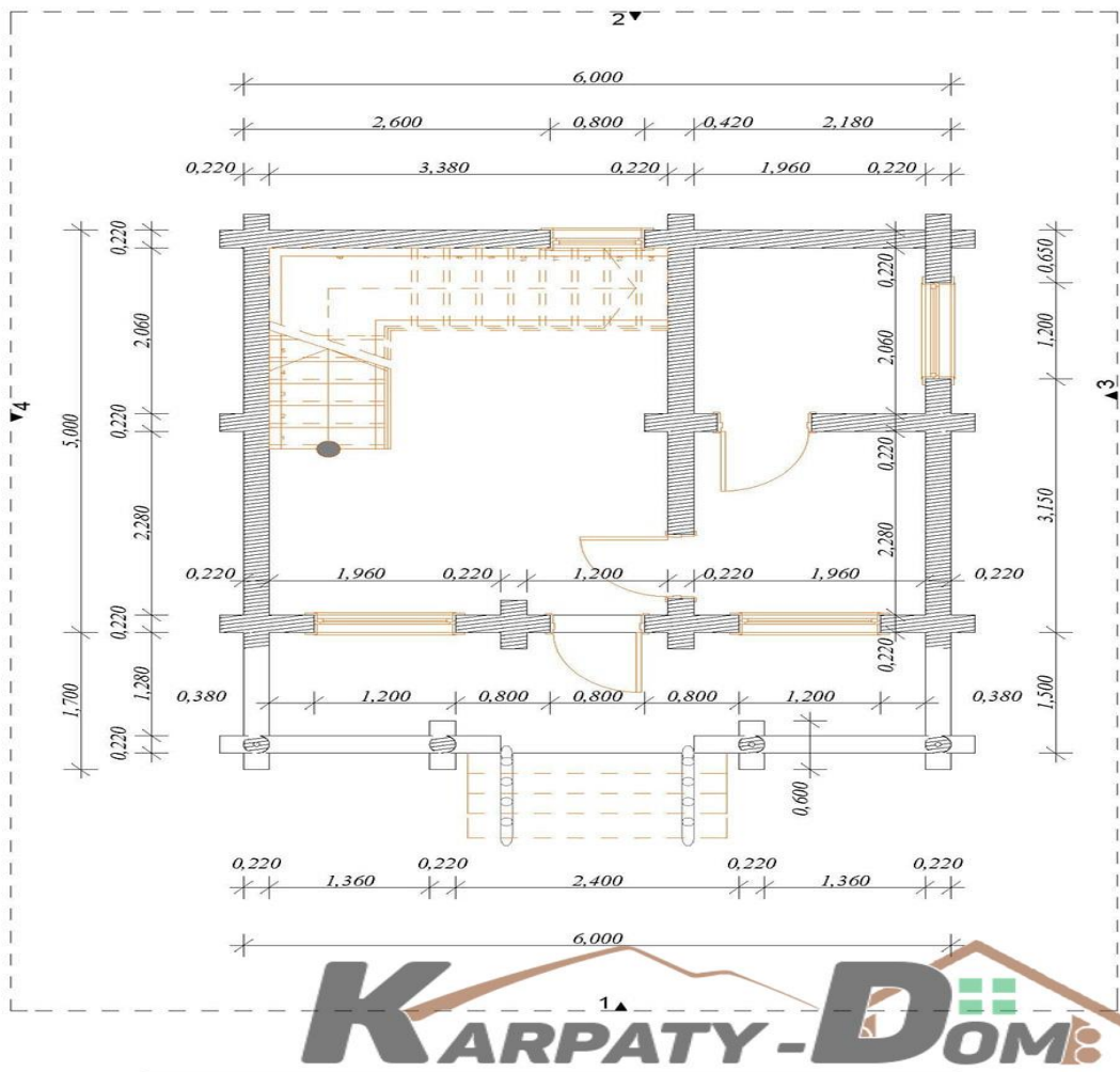
План первого поверху M 1:50
