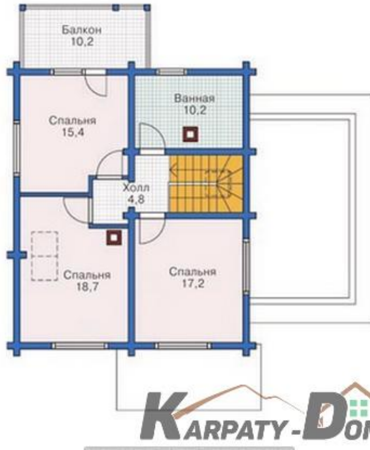
План мансардного этажа
