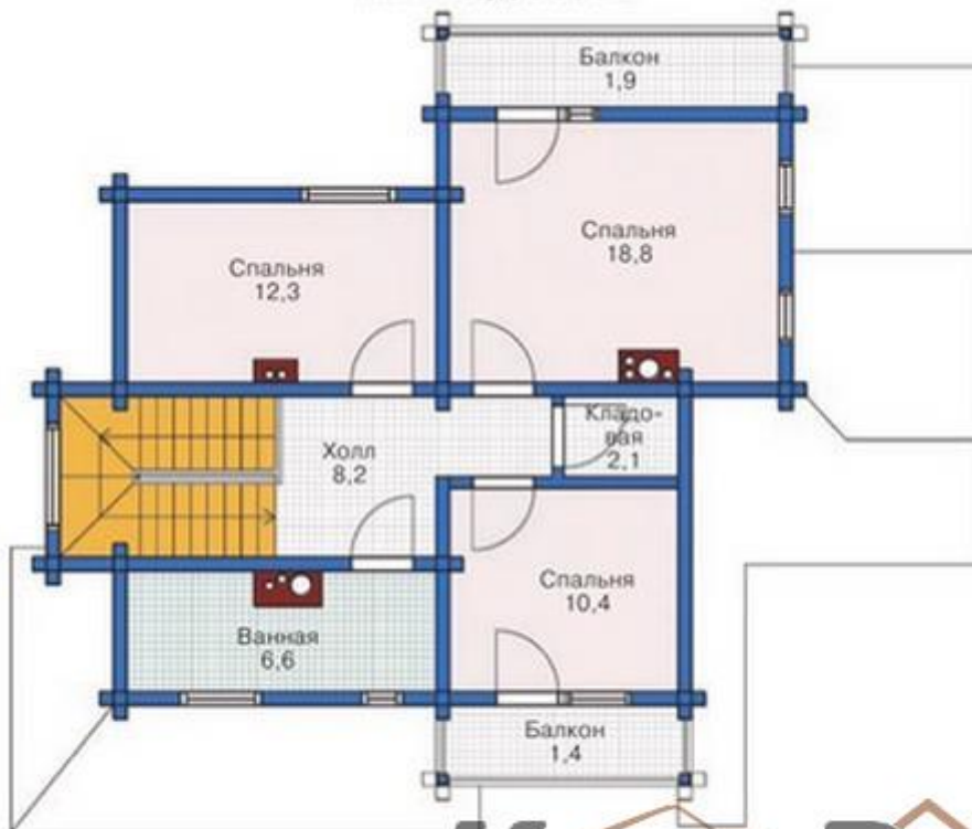
План мансардного этажа
