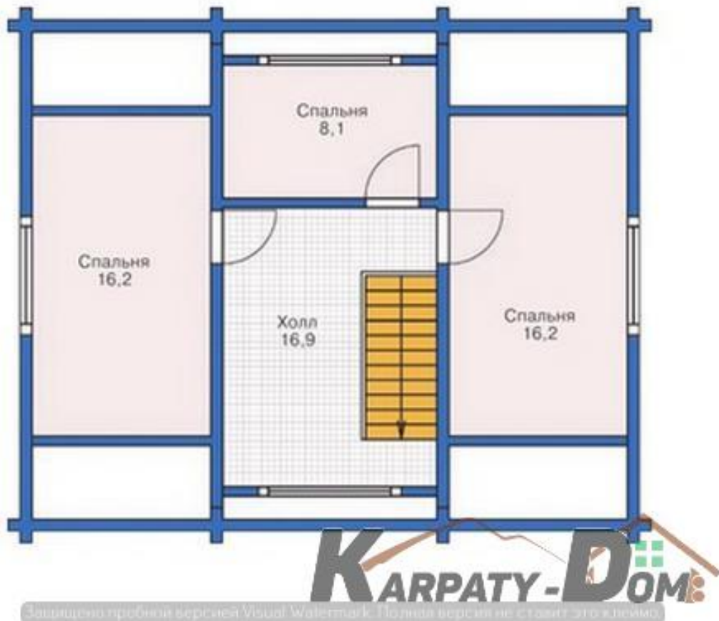
План мансардного этажа
