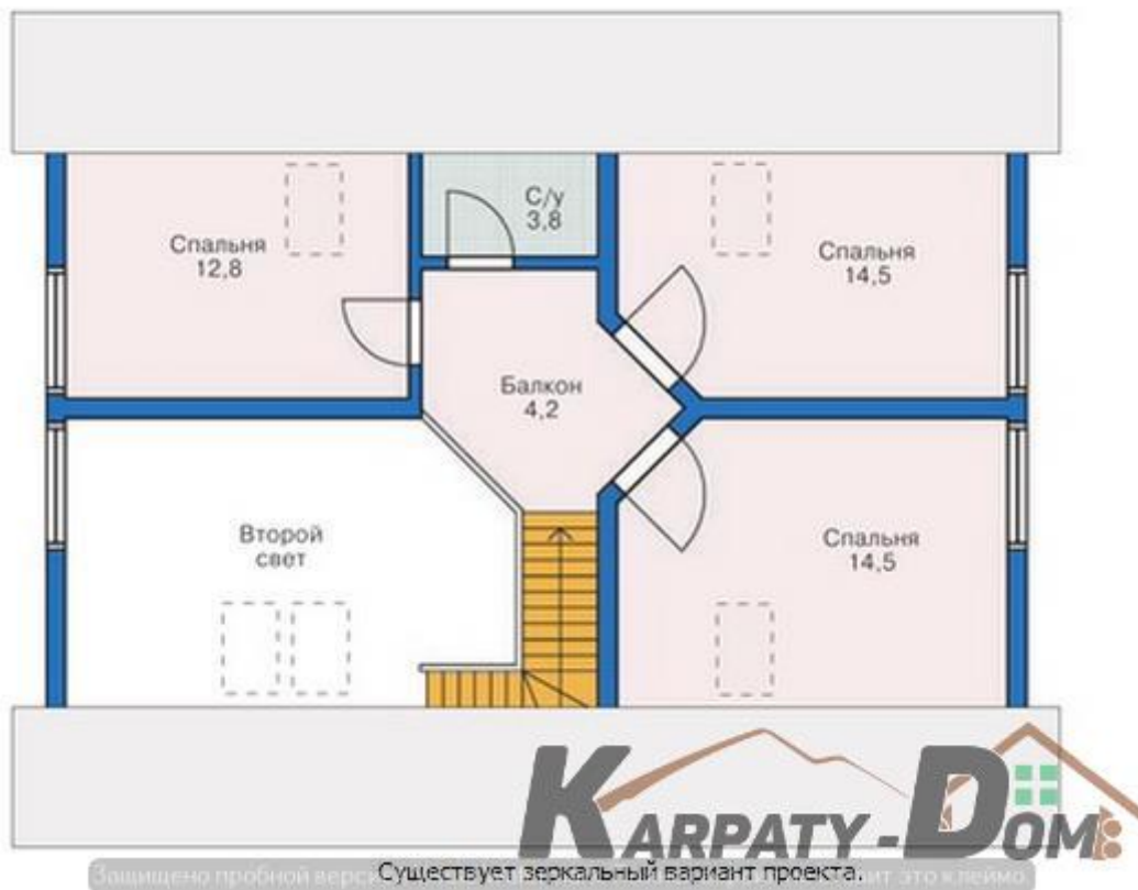
План мансардного этажа
